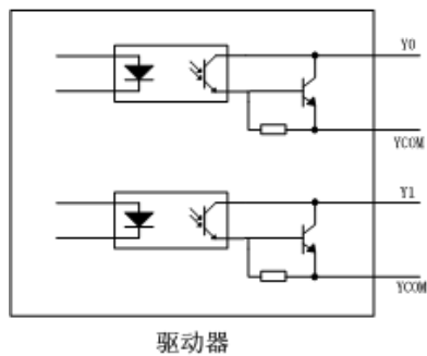
Y0-Y1 输出端子内部电路
