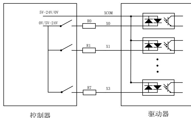
输入端子接法参考电路
