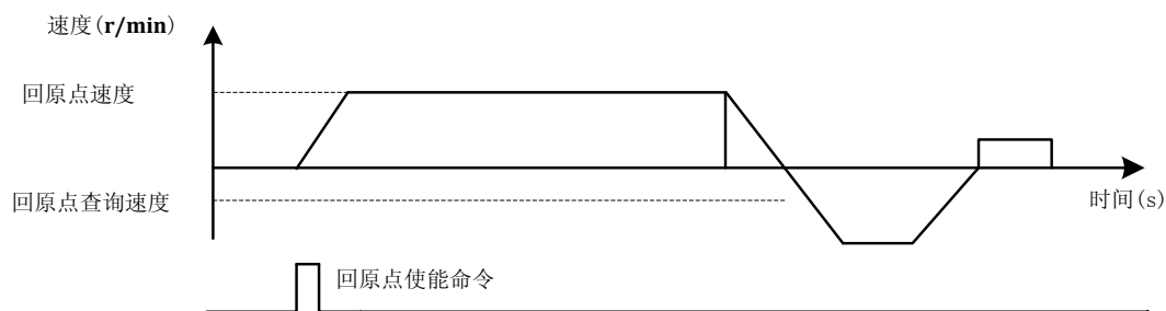
限位+补偿回原点工作流程
