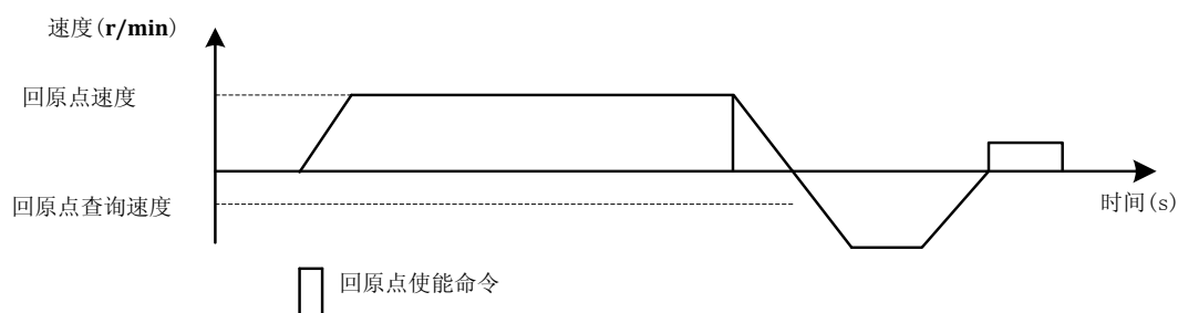
限位+原点回原点示意图
