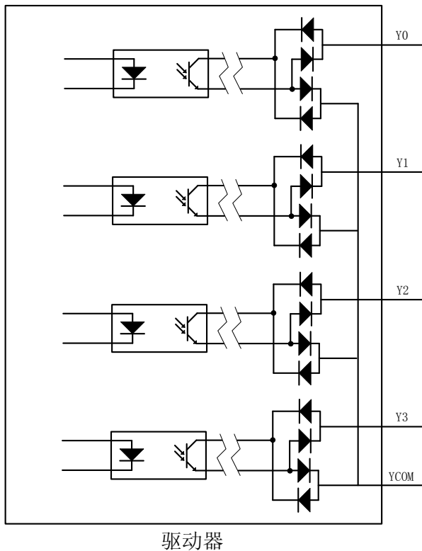
Y0-Y3 输出端子内部电路
