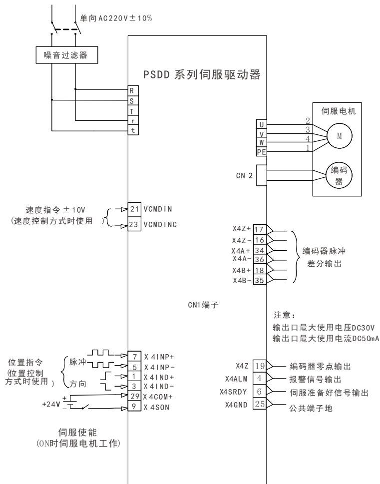
• 使用外部电源时CN1接线图
