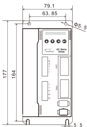
安装尺寸正面图
