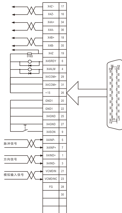
• 使用内部电源时CN1接线图
