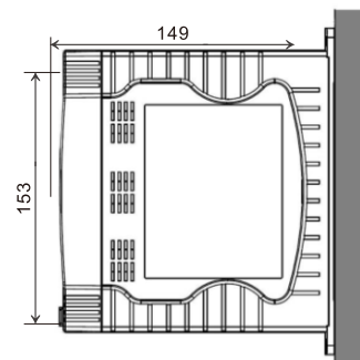
安装尺寸侧面图
