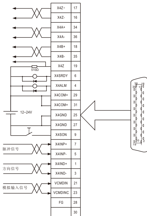
• 使用外部电源时CN1接线图
