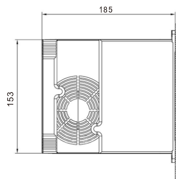
安装尺寸侧面图
