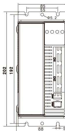
安装尺寸正面图
